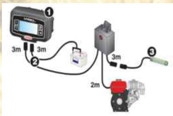
Control umplere bazin cu senzor de nivel
